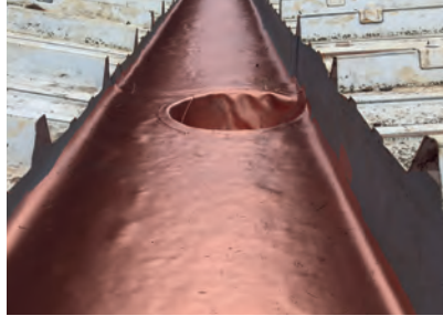
Chemisage cheneau
